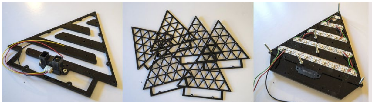
Triangle Aufbau
