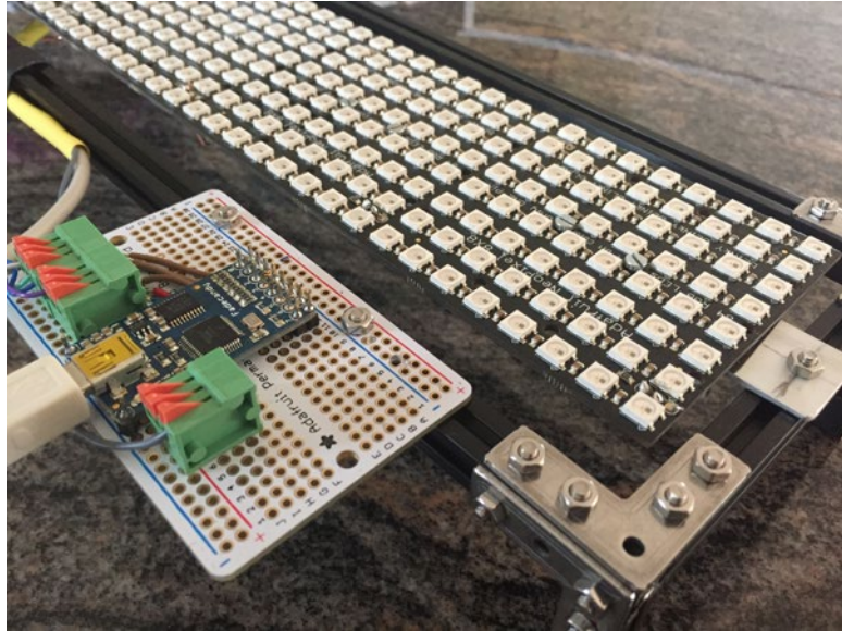
Testaufbau
